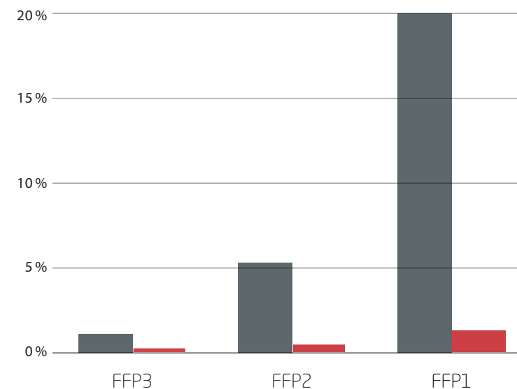
Filterleistung Partikeldurchlässigkeit
